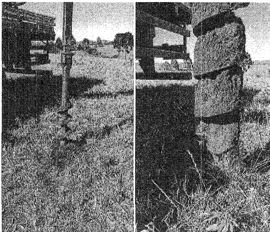
TE33- Perfuração 1: 3,10 cm de profundidade- terra cascalho
