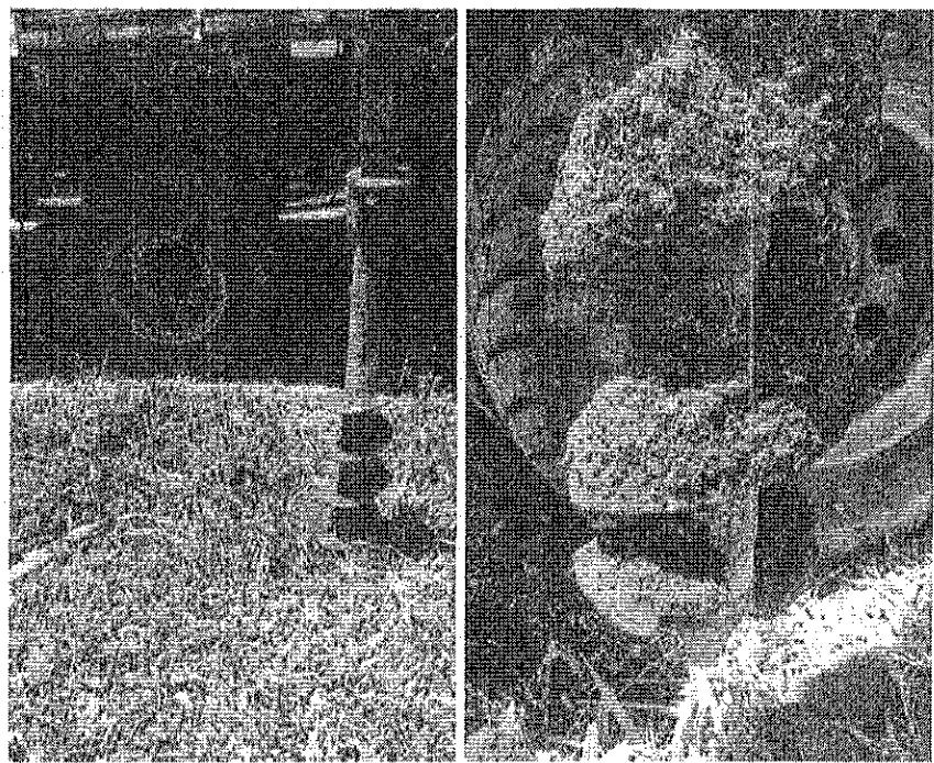
TE8-Perfuração 1: 1 m de profundidade- terra solta- laje
