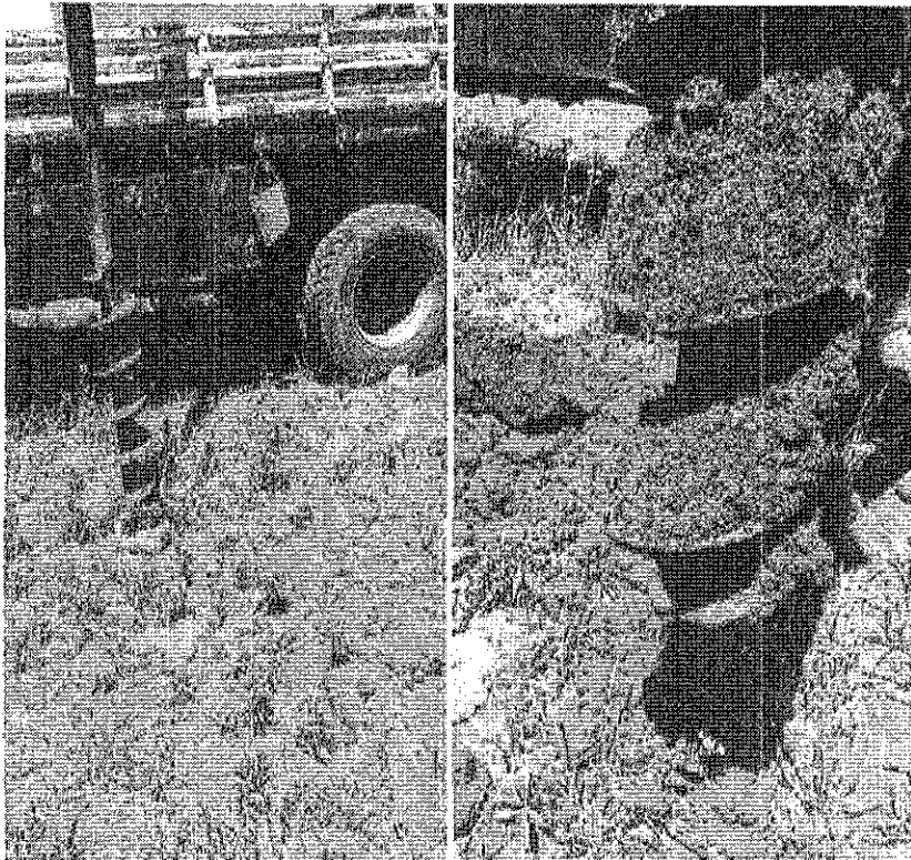
TE6- Perfuração 1: 1,10 cm de profundidade- terra rachão- laje
