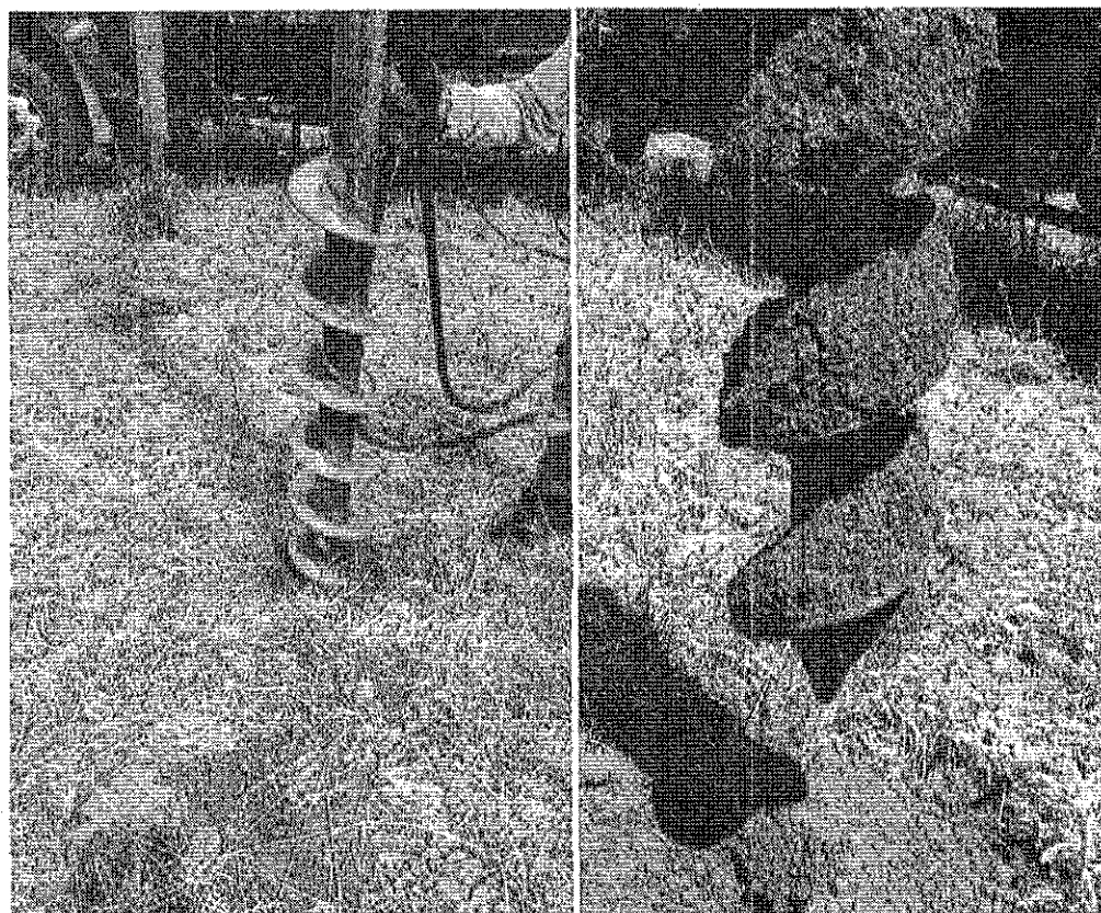
E6- Perfuração 1: 4,35 cm de profundidade- terra cascalho
