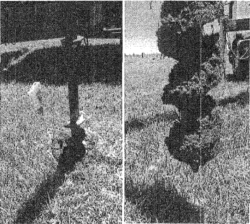
TE8-Perfuração 1: 1 m de profundidade- terra solta- laje
