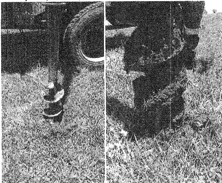
TE12- Perfuração 1: 1,80 cm de profundidade- terra cascalho- laje Perfuração 2: 1,10 cm de profundidade- terra cascalho- laje
