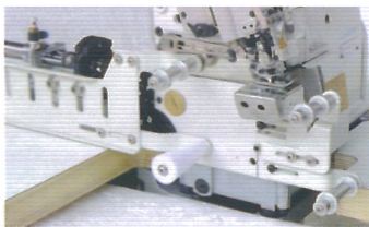
Optional: rolete (fixo ou móvel) para aplicação de elástico
