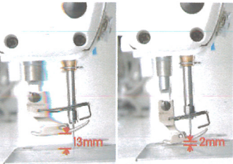
Acionamento do calcador por motor de passo.
